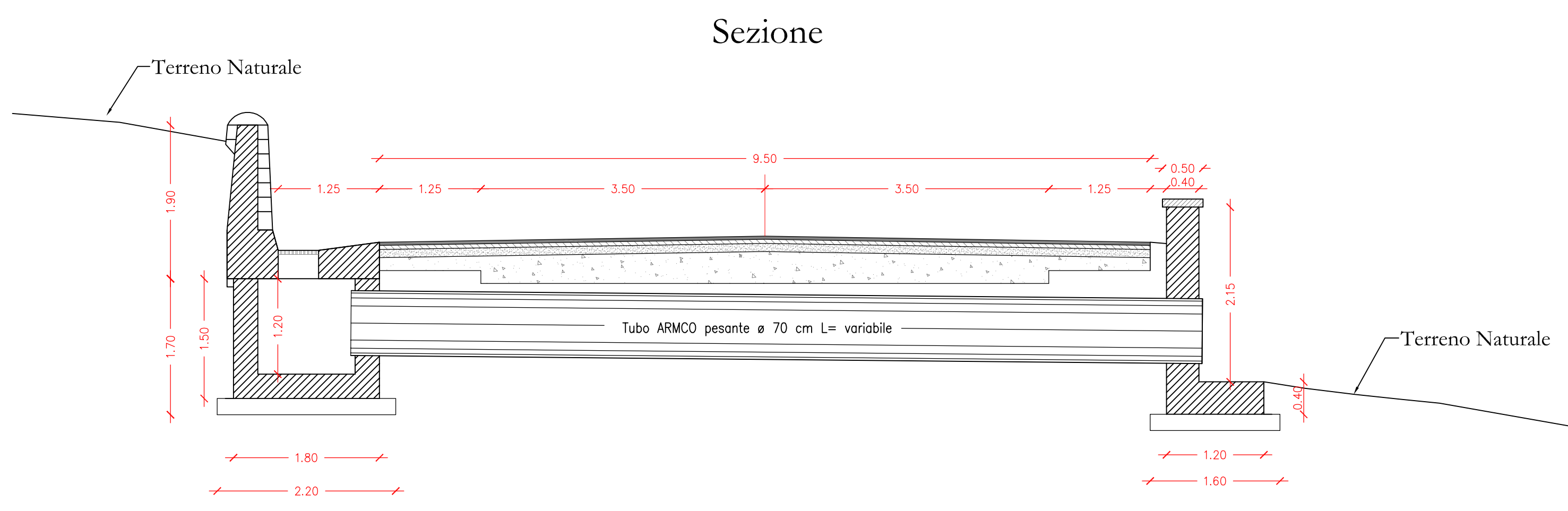
Tombino Tubazione in ARMCO \phi 70 CM scala 1:50
